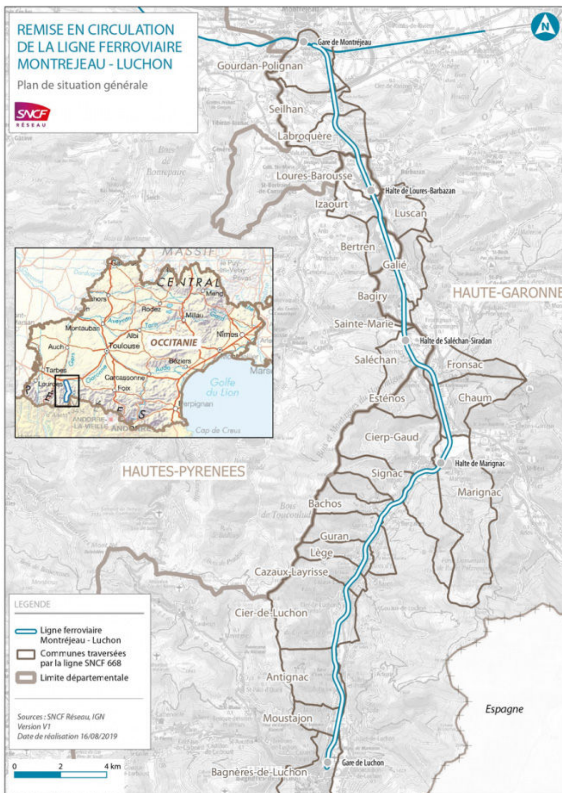
Fig. 15 : Plan du projet de tracé de la ligne ferroviaire et des arrêts envisagés dans la vallée de la Garonne (source SNCF réseau)
